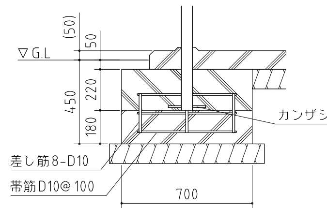
A-A' 断面 1/20
